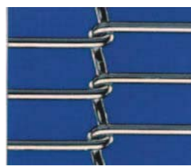
Paso 9,6 mm Ø 2,08 mm
