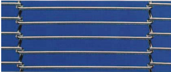
Paso 6 mm Ø 1,27 mm
