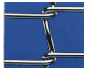
Paso 20,32 mm Ø 2,34 mm
